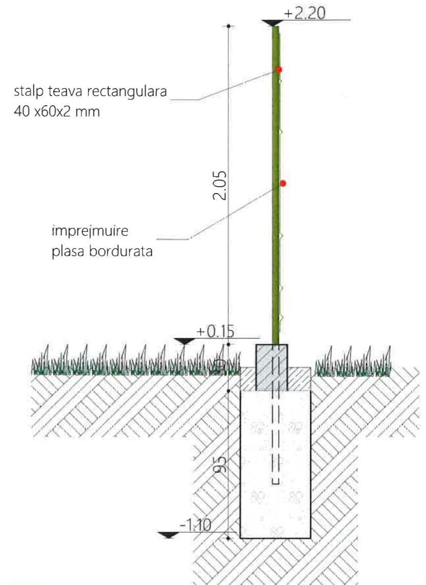
sectiune transversala
