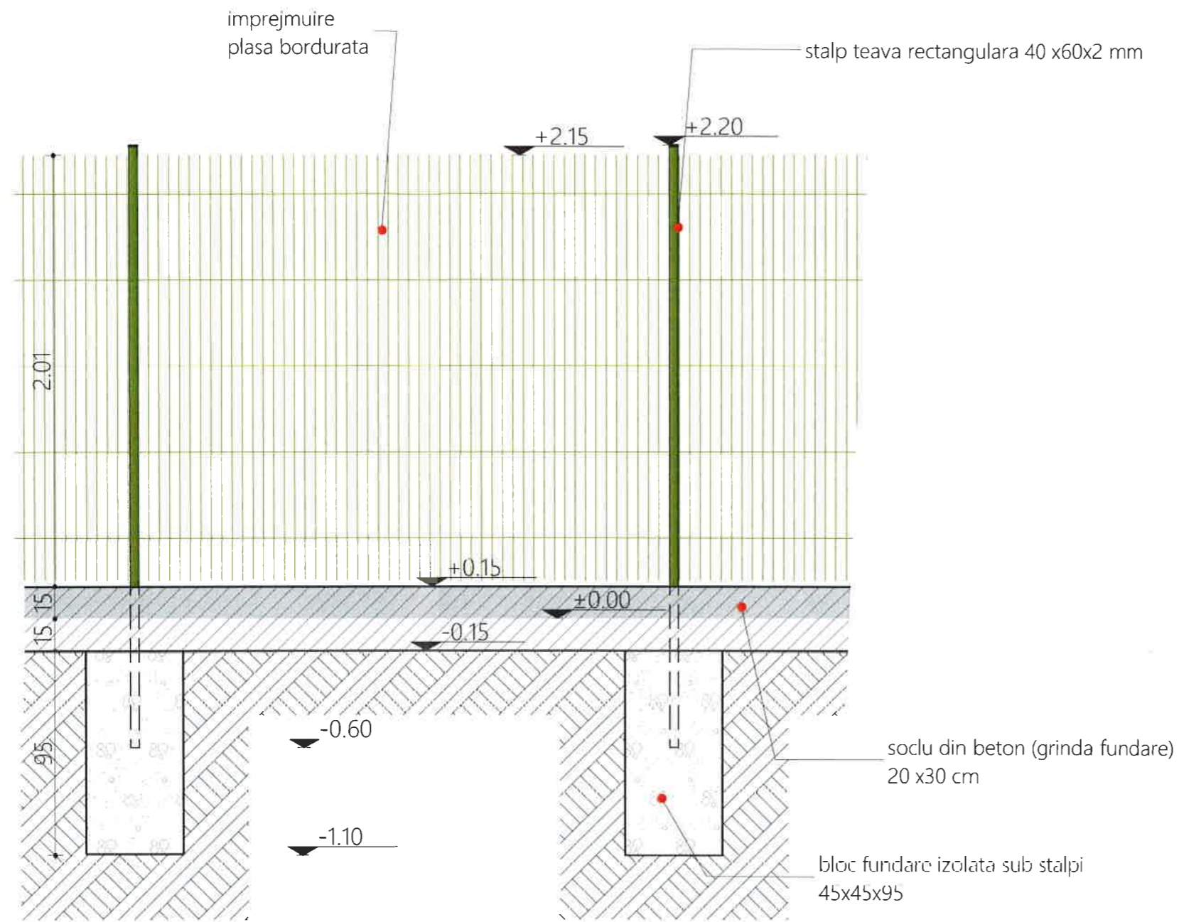
sectiune longitudinala
