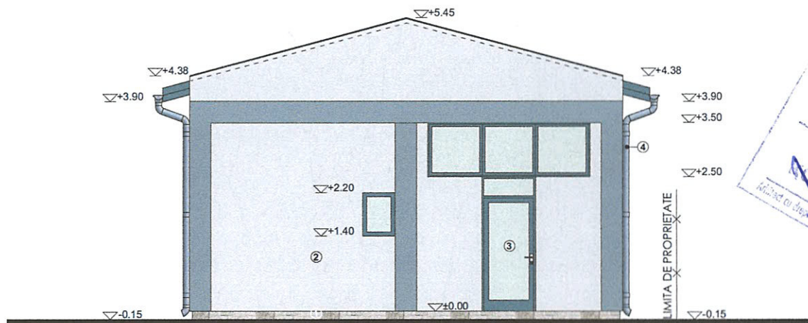
FATADA POSTERIOARA
